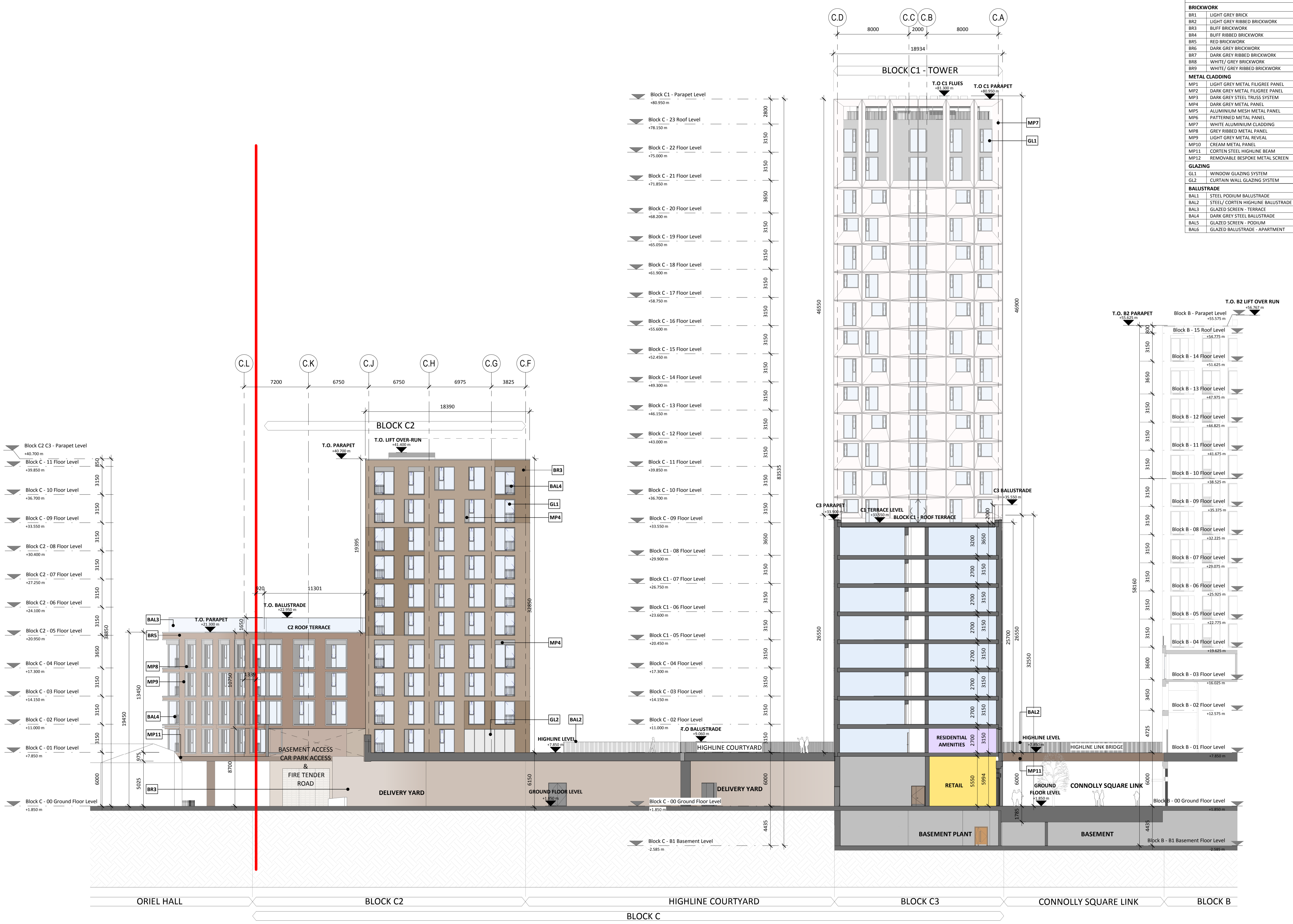
02 BLOCK C - SECTION 02 1 : 200
