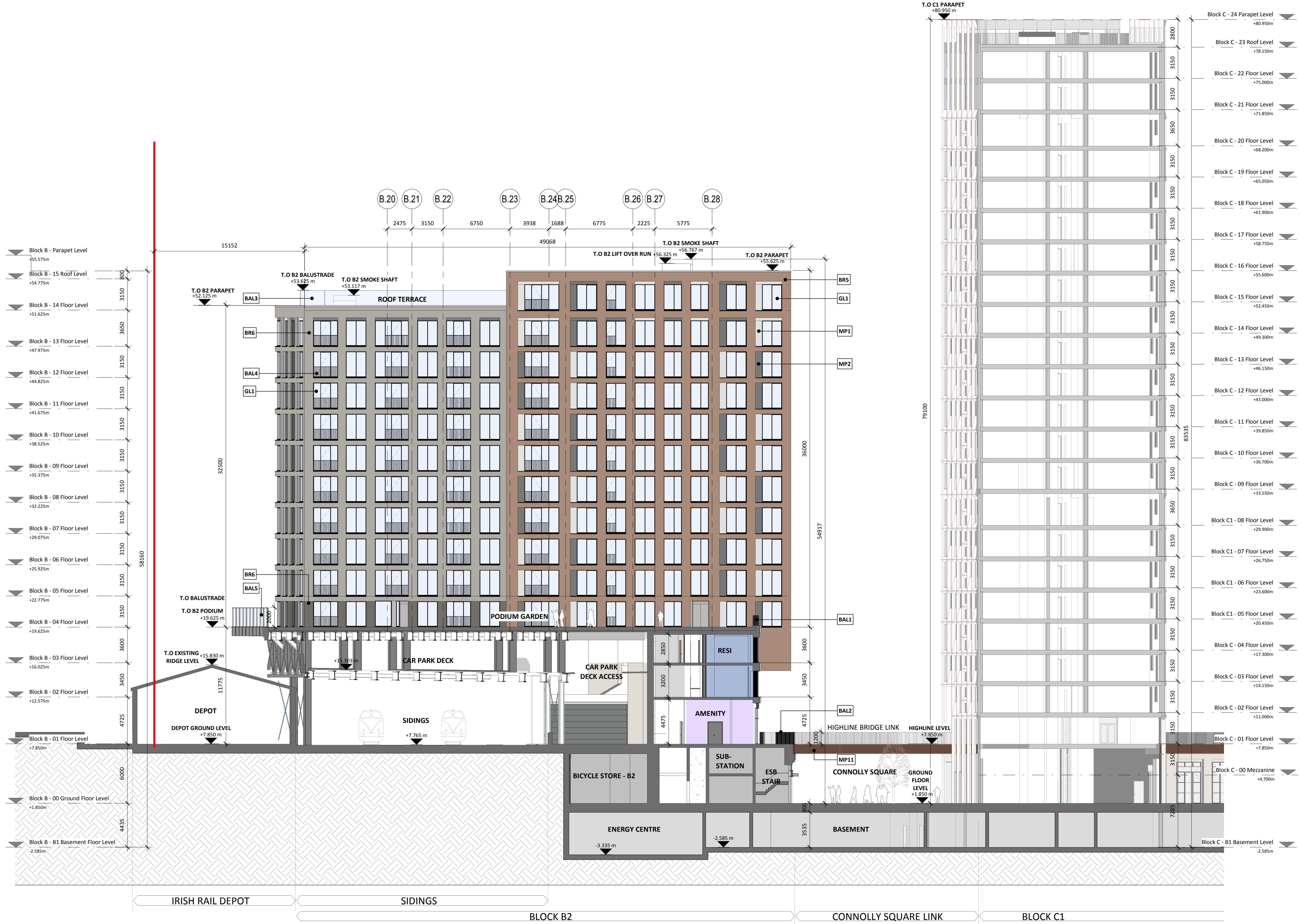
D-D BLOCK B - SECTION D-D 1 : 200
